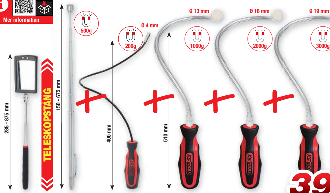
550.1090 Flexibel och teleskopisk magnethållare och inspektionsspegelset
