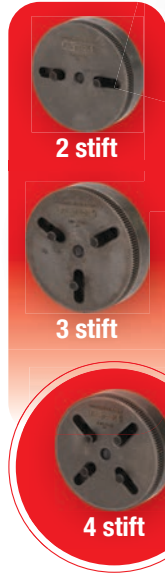
150.2440 Universal bromskolv-återställnings-verktyg-sats
