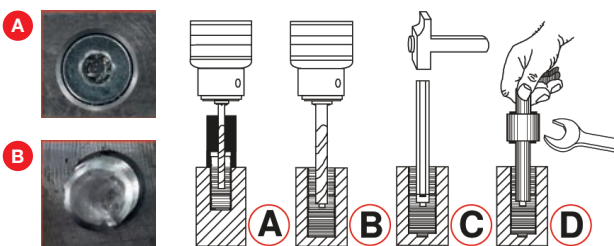
150.1305 M5 - M6 - M8 - M10 - M12 - M14 - M16 Skruvutdragning-sats
