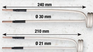
500.8680 Induktionsvarmluftspistol-sats
