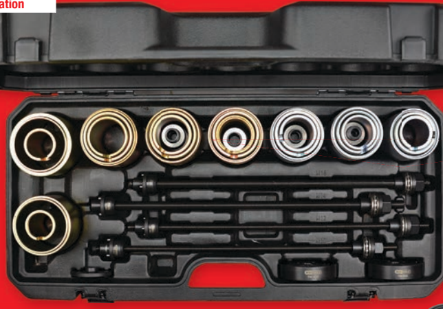
700.1550 Tryck-och draghylsesats
